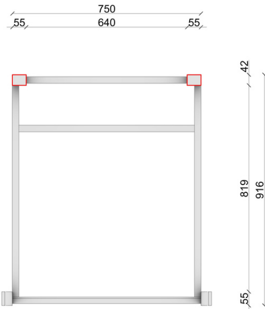
PRZEKRÓJ CC
