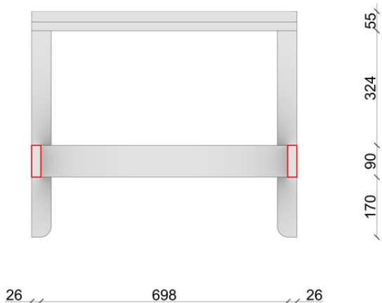
PRZEKRÓJ CC
